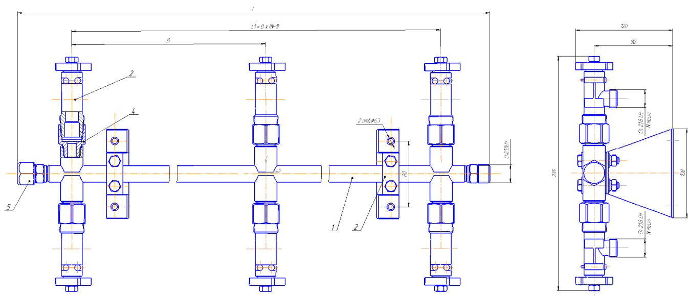
Рис.1 Коллектор рамповый КР-03 ДЖЕТ 305 35 00 00
